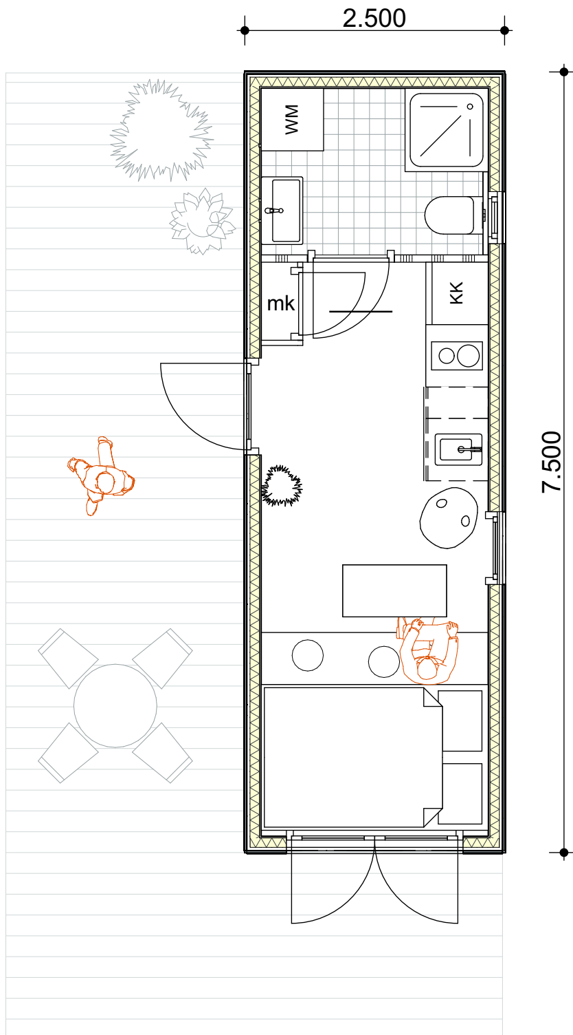
plattegrond schaal 1:50
